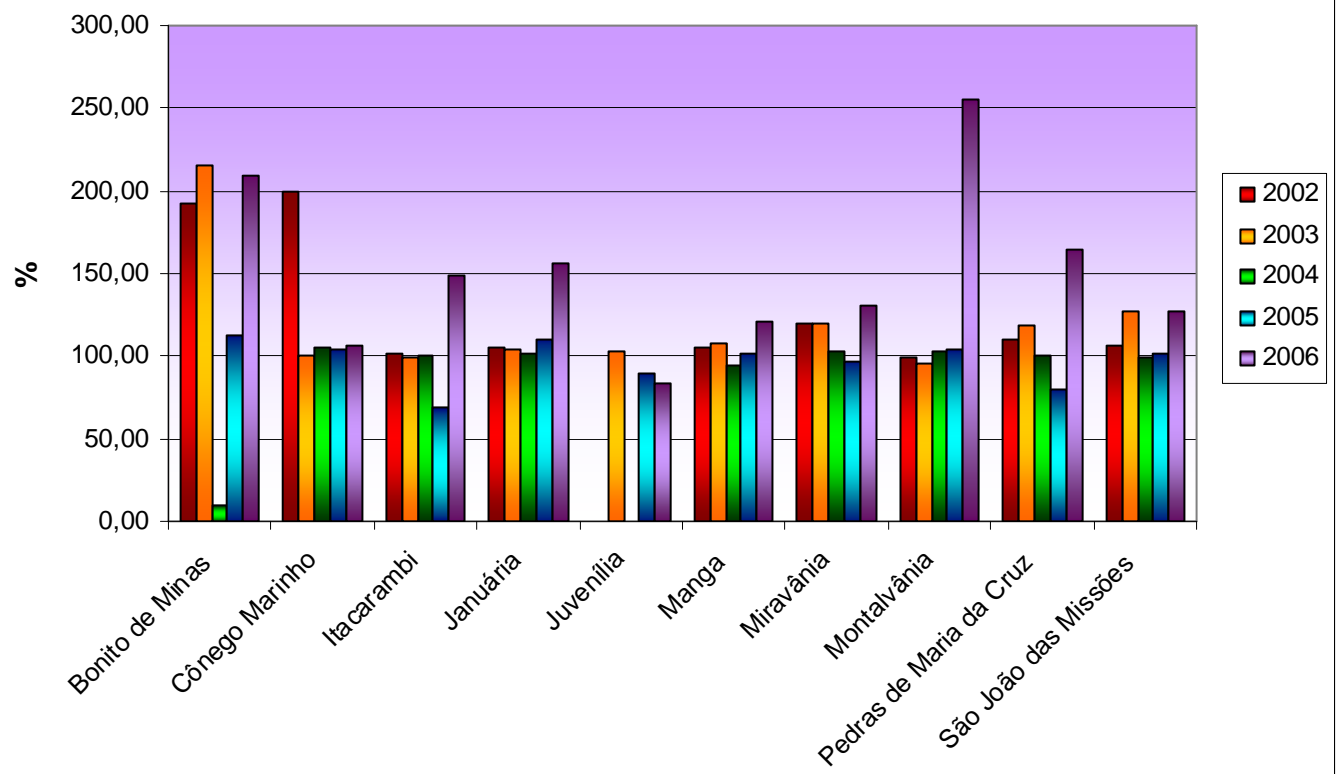
Percentual de imóveis vistoriados na atividade de tratamento focal e tratamento vetorial, Microrregião de Januária, Minas Gerais 2002 - 2006
